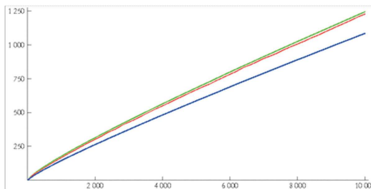
Figura 1: Gráficos de \pi(x) (a vermelho), \int_0^x \frac{1}{\log t} dt (a verde) e x/\log x (a azul)
